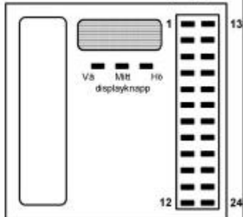
DCS24B med display
